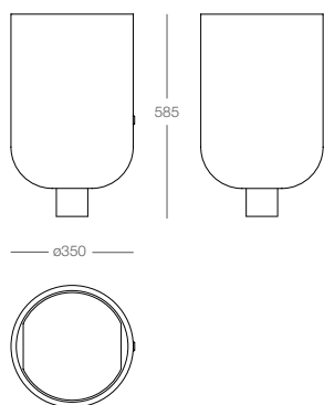
litter bin 32L corbeille 32L papelreira 32L
