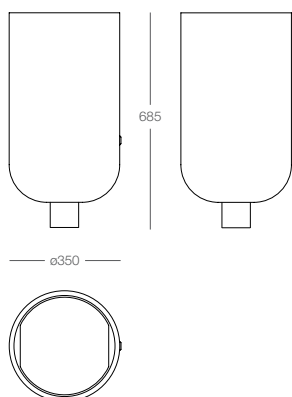
litter bin 42L corbeille 42L papelreira 42L
