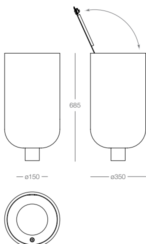
litter bin with lid 42L corbeille avec couvercle 42L papelreira com tampa 42L
