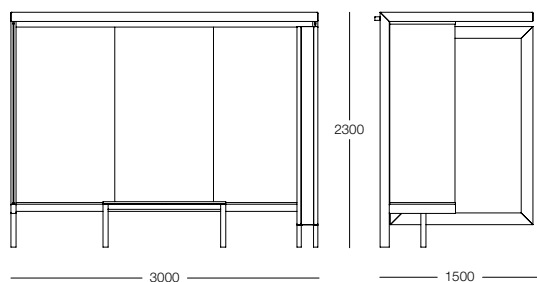
shelter with mupi abribus avec mupi abrigo com mupi
