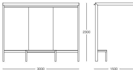
shelter (with optional bench) abribus (avec banc optionnel) abrigo (com banco opcional)
