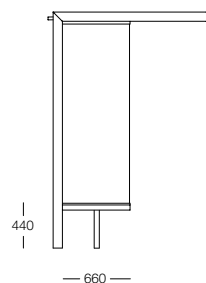
shelter with side panel abribus avec panneau latéral abrigo com painel lateral
