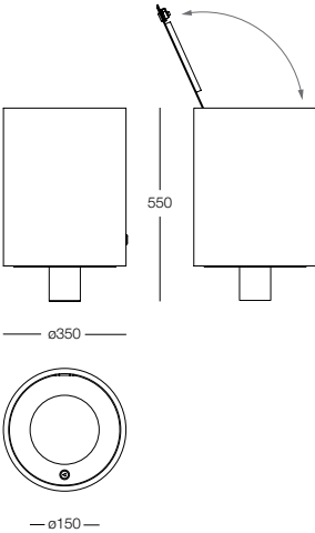
litter bin with lid 32L corbeille avec couvercle 32L papeleira com tampa 32L
